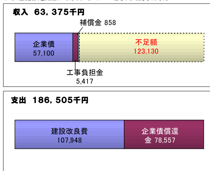
図2 資本的収支
