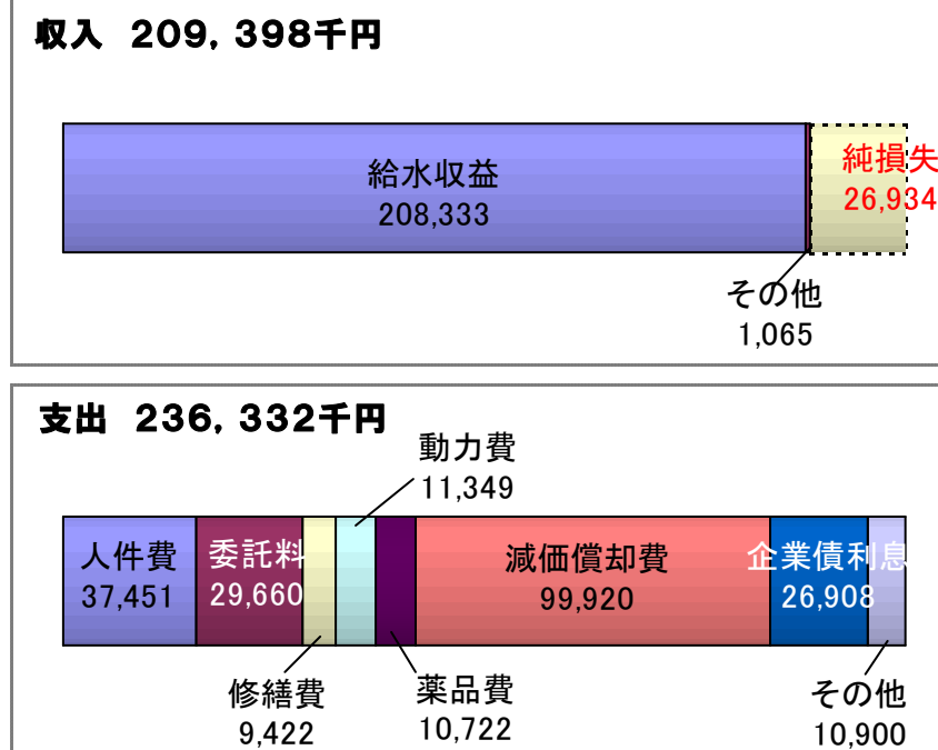
図 1 収益的収支
